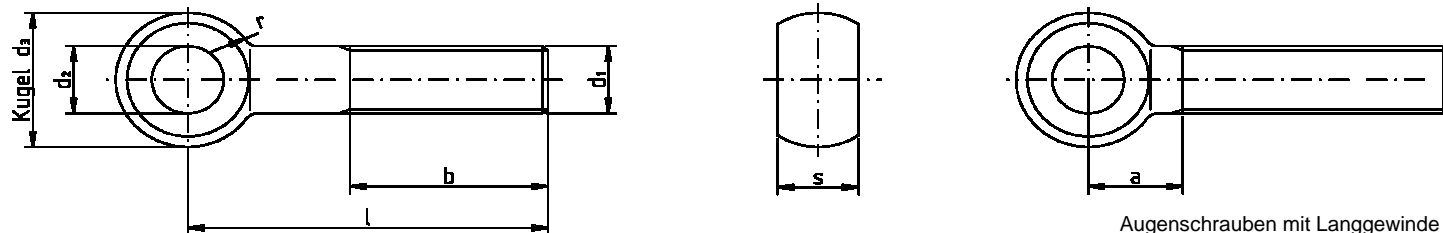
Augenschrauben mit Langgewinde
